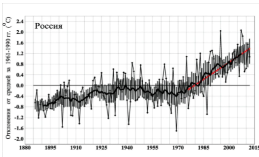
Рис. 22. Изменения аномалий среднегодовой температуры приземного воздуха на территории России в 1886–2012 гг. Источник: Росгидрометр
