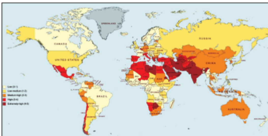
Рис. 10. Отношение объема потребления пресной воды к объему доступных возобновляемых источников. Источники к: составлено авторами на основе данных Baseline Water Stress, World Resource Institute
