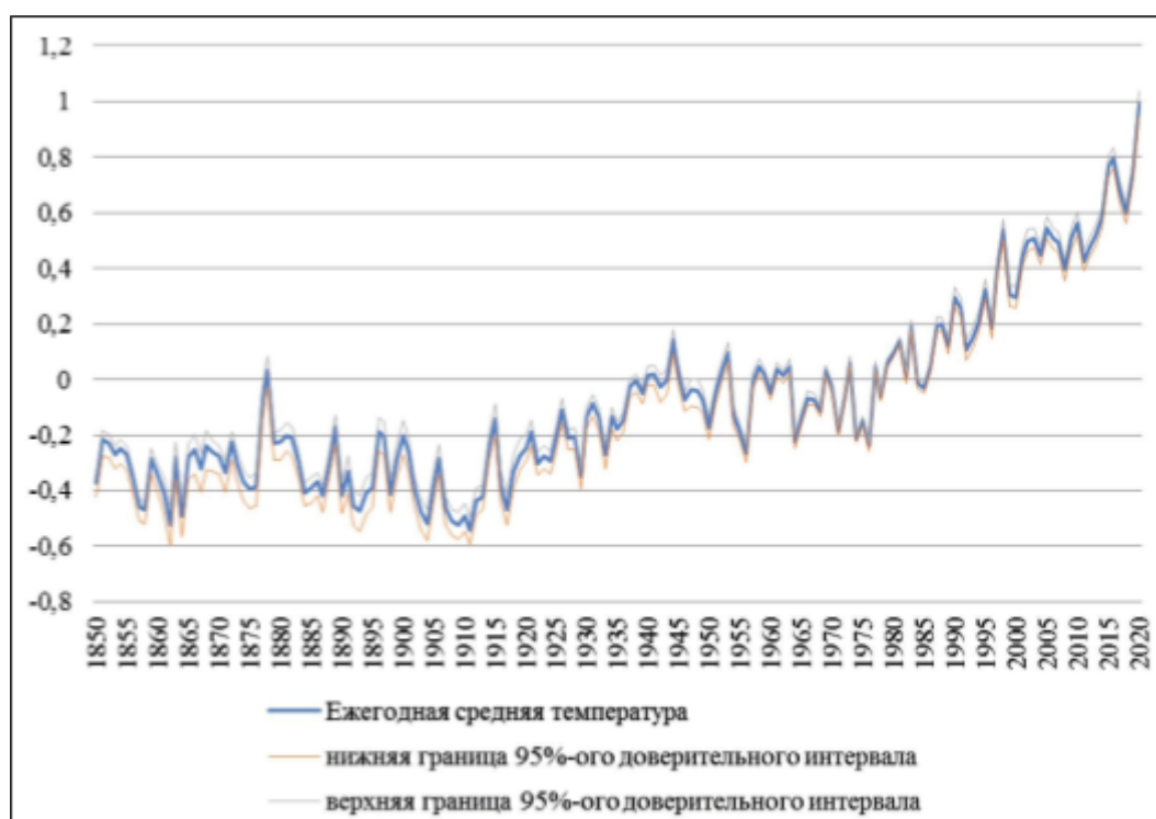
Рис. 11. Отклонение средней приземной температуры Земли в 1980–2019 гг. от средней за 1961–1990 гг., °C. Источники: Met Office Hadley Centre for Climate Science and Services
